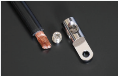
4ゲージ電源ケーブルをターミナルから外した時の導体画像である。導体全体が均一に圧着された理想的な導体。
