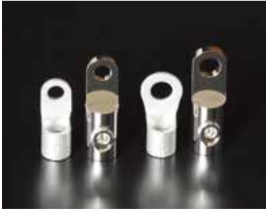
M&M DESIGN製ロジウムターミナルと裸圧着端子との比較画像。
